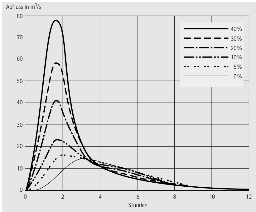
Grafik Nr. 4: Abflußganglinien bei gleichem Niederschlag unterschiedlichem Versiegelungsgrad (0 bis 40 %), Einzugsgebiet 20 km 2
